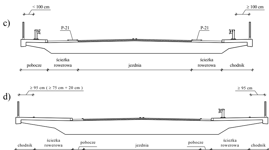
Rys. 7. Chodnik na obiekcie mostowym - przykłady.
