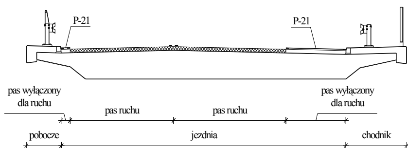
Rys. 3. Pasy wyłączone dla ruchu wyznaczone na jezdni - przykłady.
