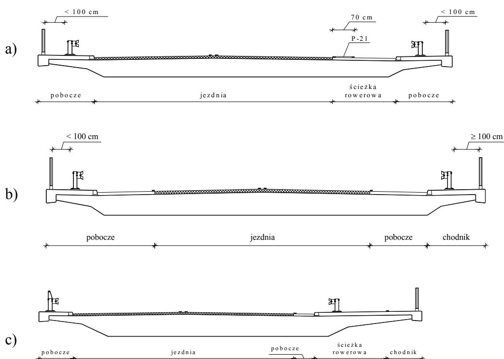
Rys. 4. Pobocze na obiekcie mostowym - przykłady.
