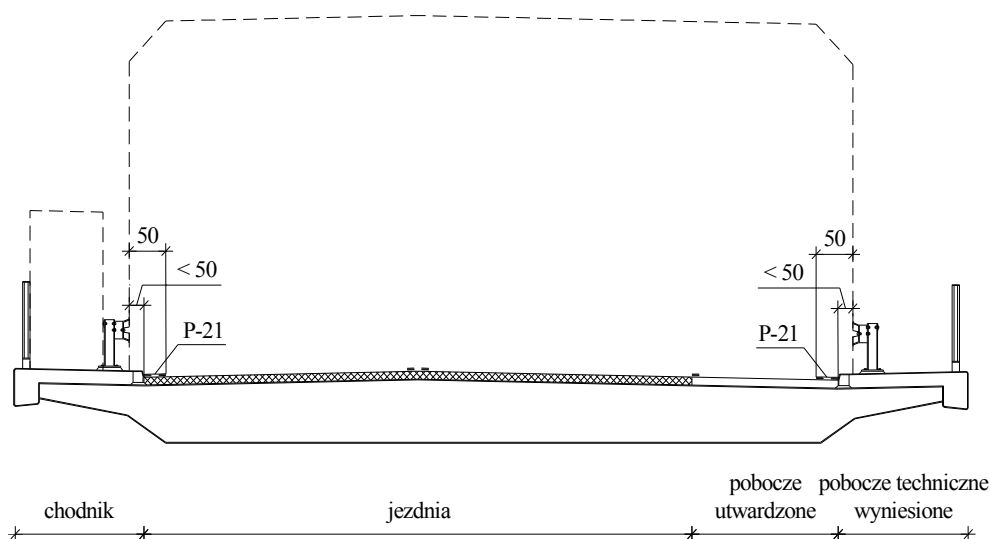
Rys. 16. Schemat skrajni drogi na obiekcie mostowym – przypadek szczególny usytuowania pasów bezpieczeństwa.
