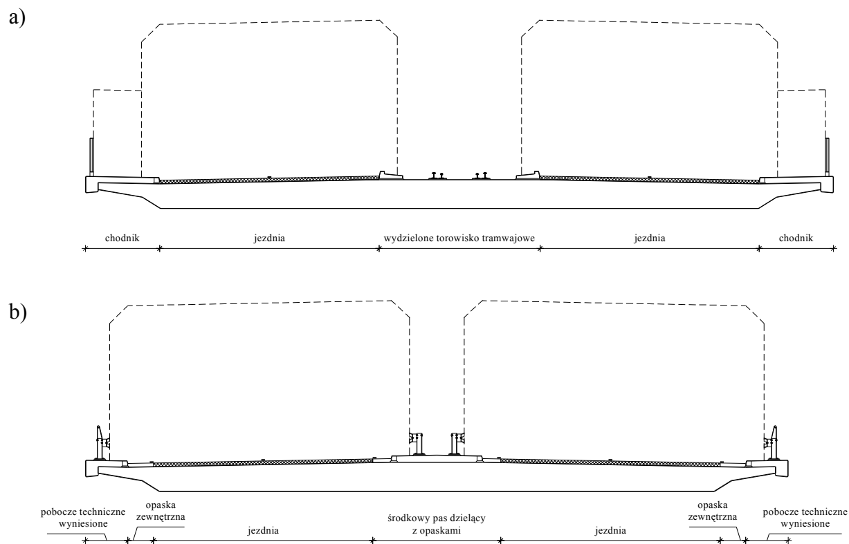
Rys. 19-3. Skrajnie drogi i chodnika na drodze dwujezdniowej, w przekroju poprzecznym obiektu mostowego.
