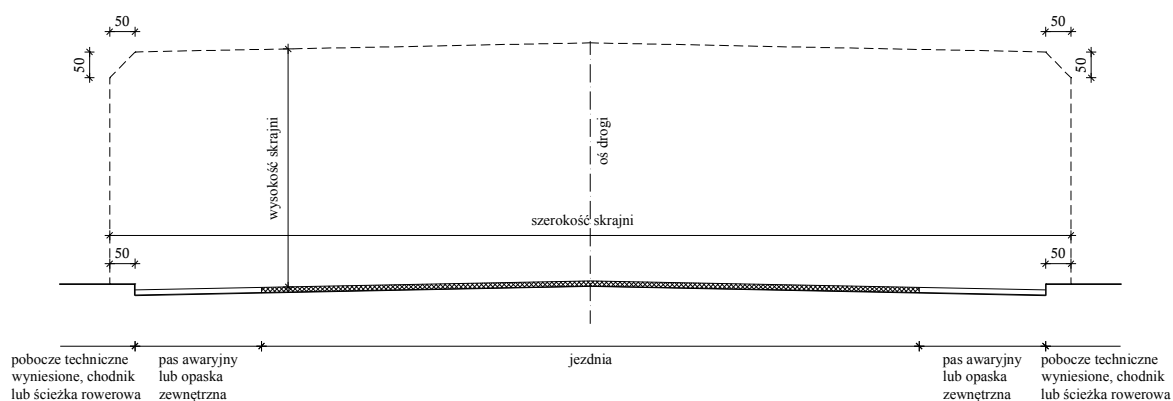
Rys. 14. Schemat skrajni jednojezdniowej drogi klasy S na obiekcie mostowy.
