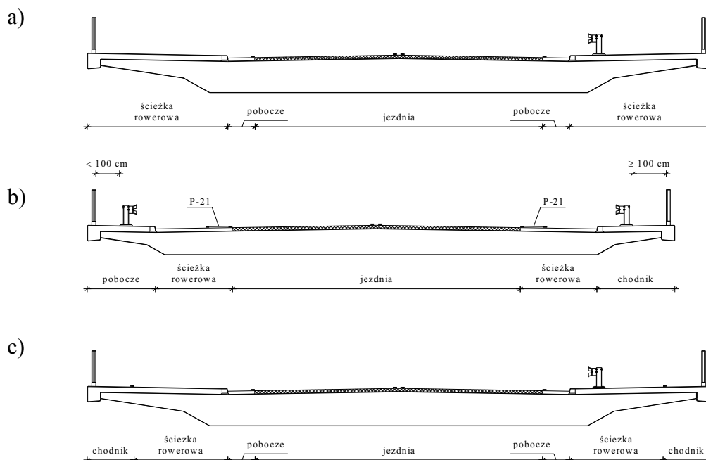
Rys. 8 Ścieżka rowerowa na obiekcie mostowym – przykłady.
