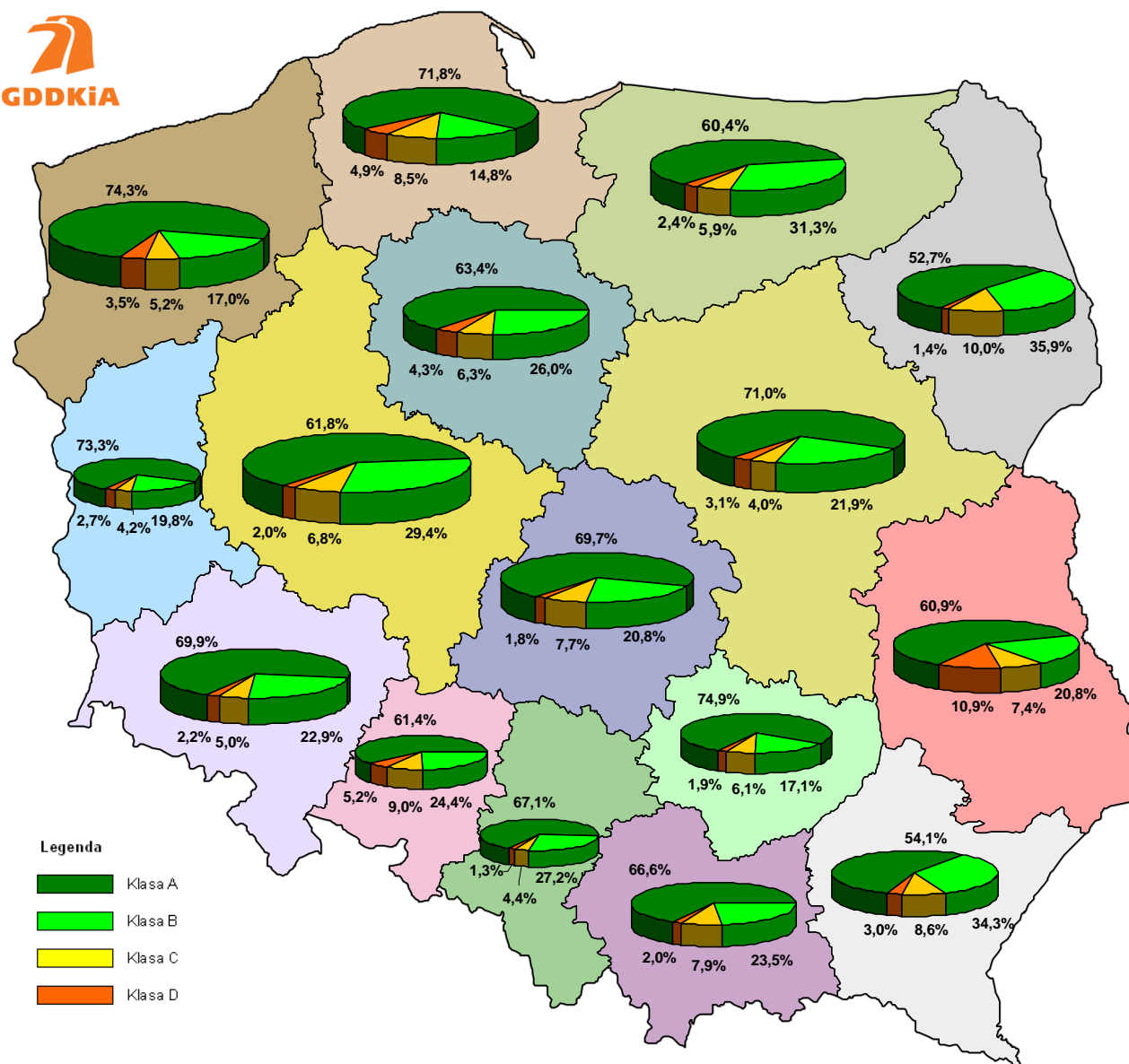
Rysunek 2. Stan techniczny parametru: równość podłużna
