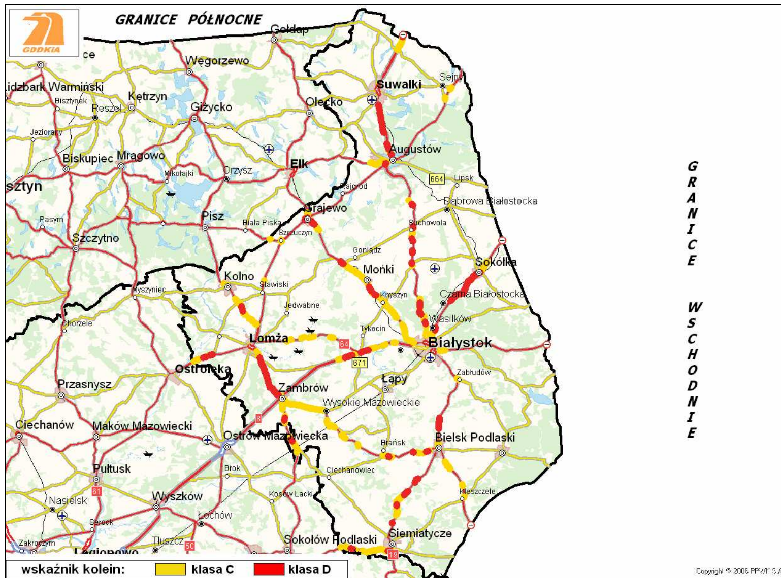
Rysunek 1. Lokalizacja odcinków dróg z koleinami w klasie C i D na terenie Oddziału w Białymstoku
