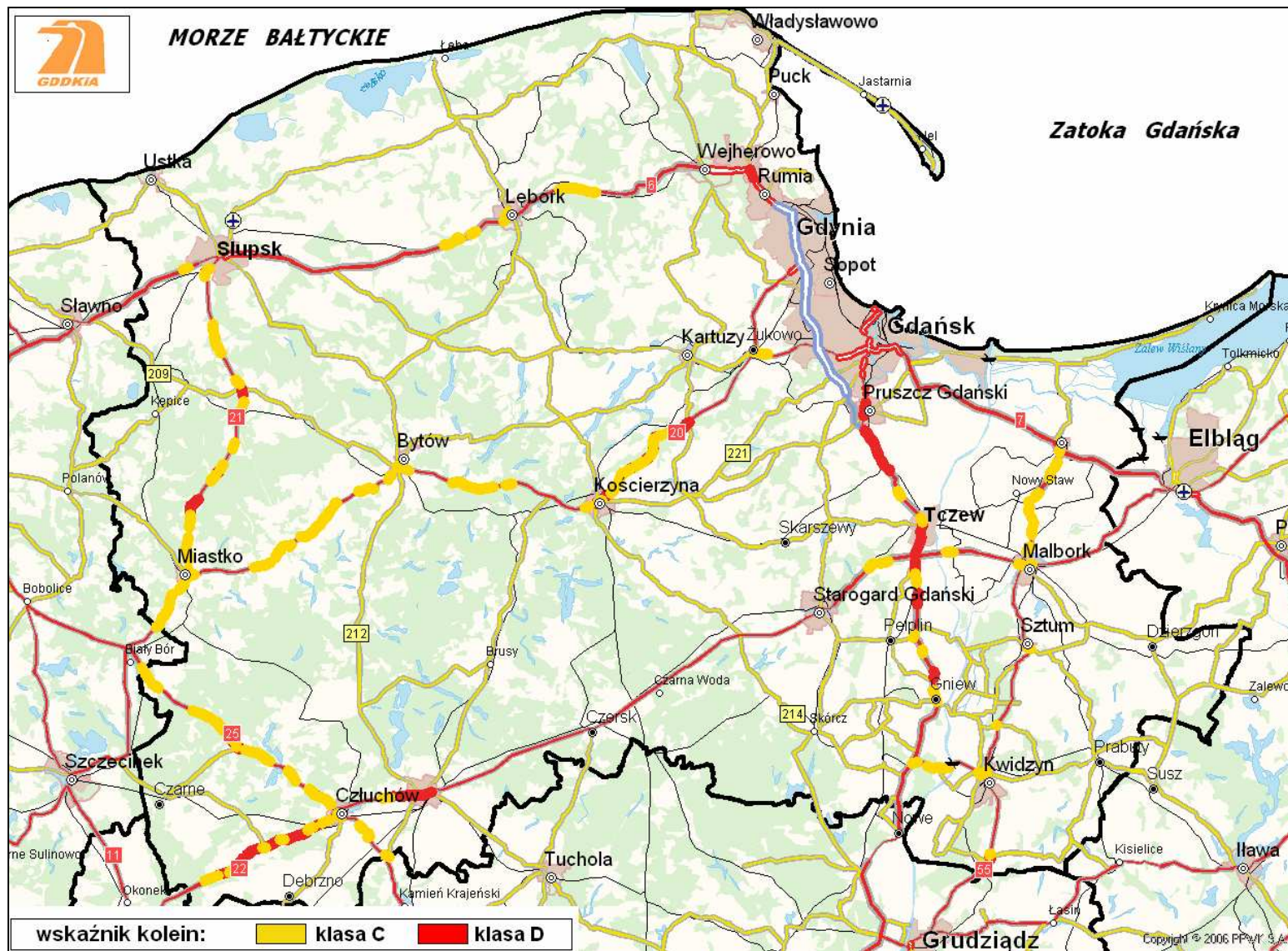
Rysunek 3. Lokalizacja odcinków dróg z koleinami w klasie C i D na terenie Oddziału w Gdańsku
