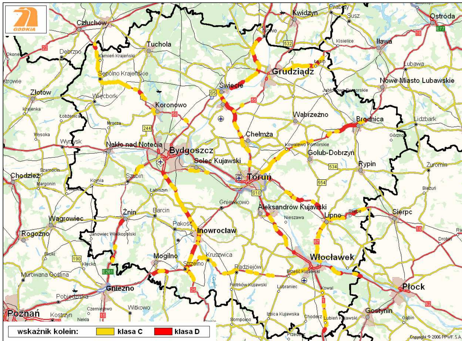
Rysunek 2. Lokalizacja odcinków dróg z koleinami w klasie C i D na terenie Oddziału w Bydgoszczy
