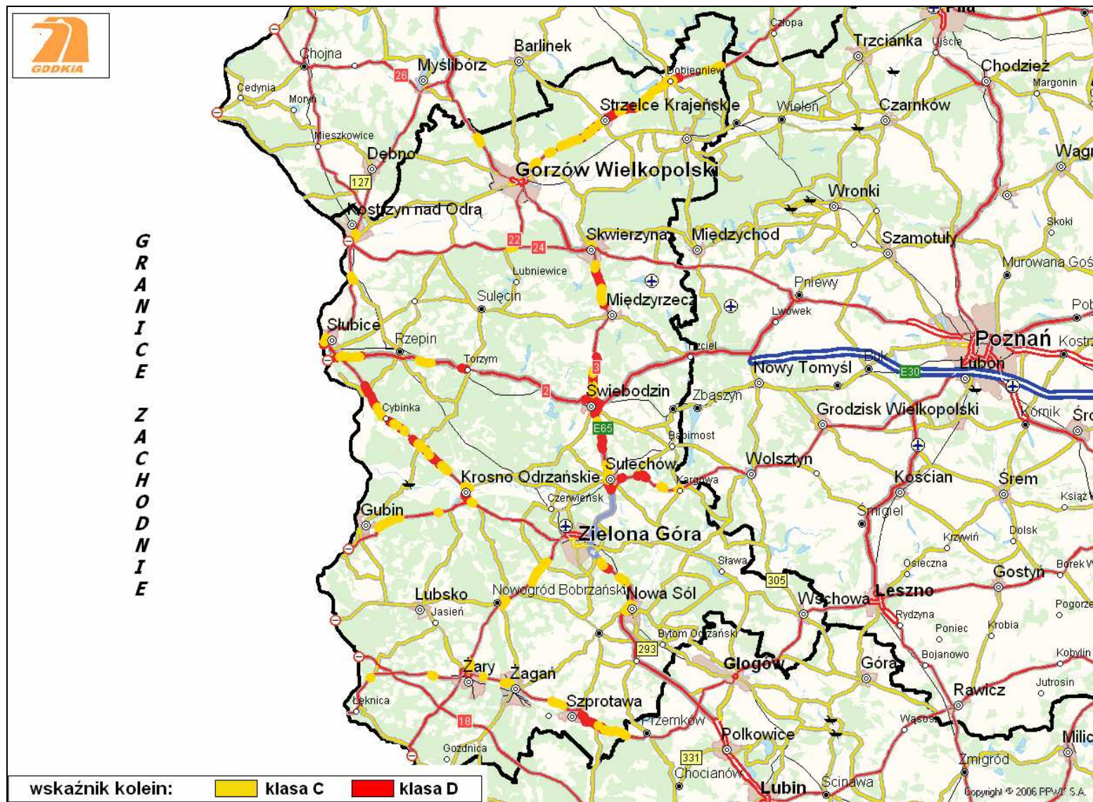
Rysunek 16. Lokalizacja odcinków dróg z koleinami w klasie C i D na terenie Oddziału w Zielonej Górze
