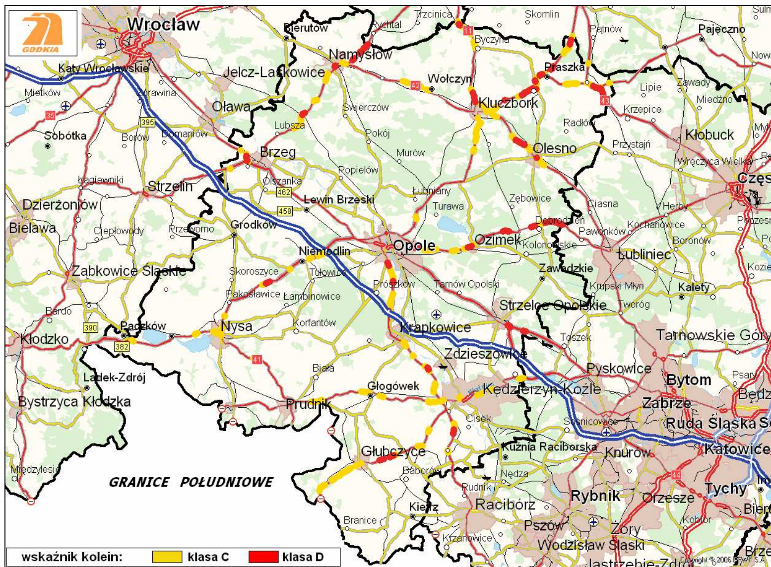
Rysunek 10. Lokalizacja odcinków dróg z koleinami w klasie C i D na terenie Oddziału w Opolu
