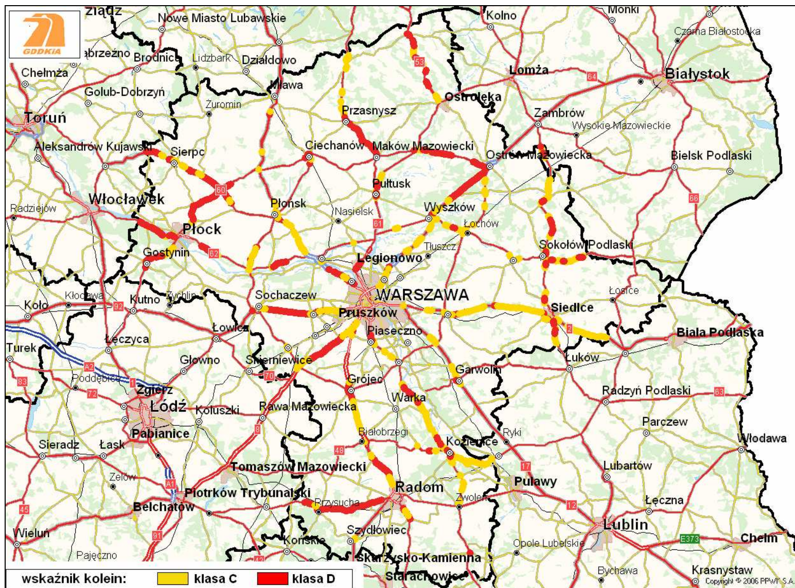
Rysunek 14. Lokalizacja odcinków dróg z koleinami w klasie C i D na terenie Oddziału w Warszawie
