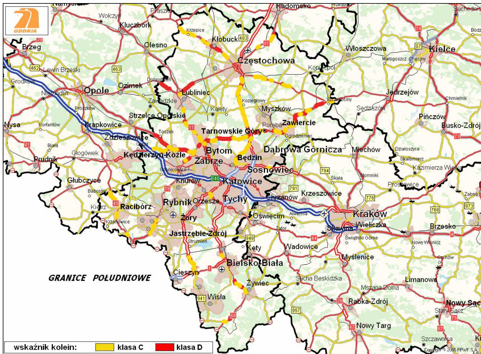
Rysunek 4. Lokalizacja odcinków dróg z koleinami w klasie C i D na terenie Oddziału w Katowicach
