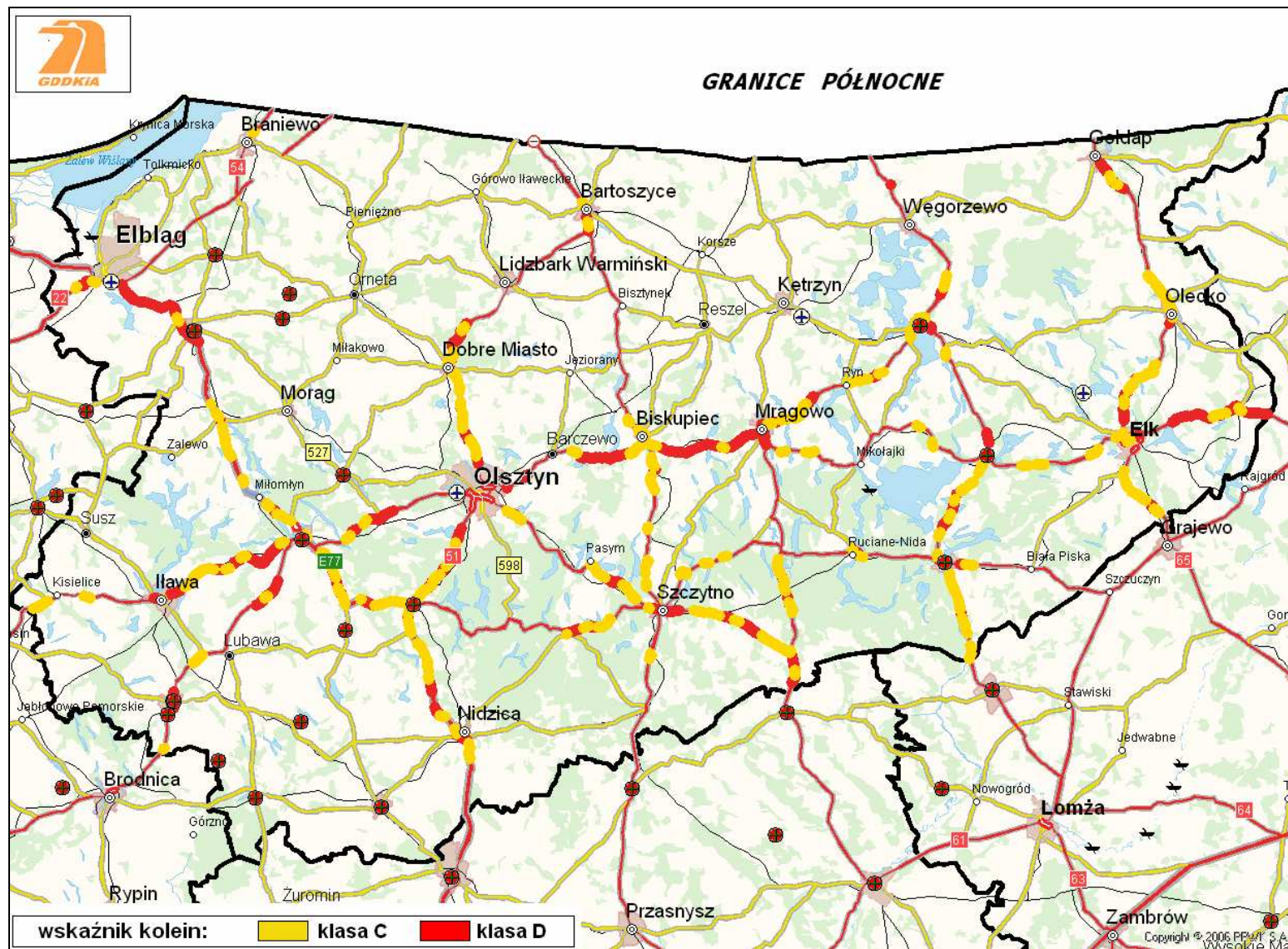
Rysunek 9. Lokalizacja odcinków dróg z koleinami w klasie C i D na terenie Oddziału w Olsztynie
