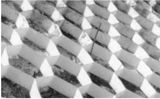
Rys. 5. Przykłady wyrobów geotekstylnych pokrewnych (geosiatki komórkowe)
