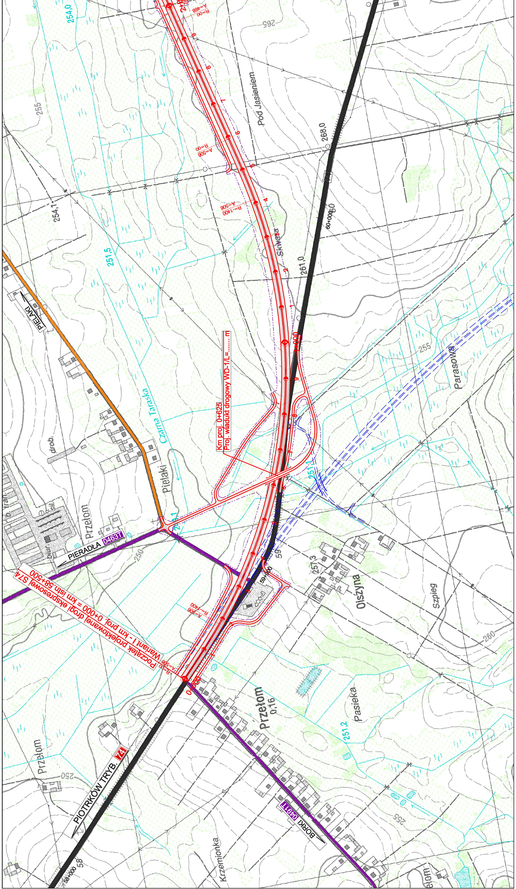
Początek projektowanej drogi ekspresowej S74 Wariant I - km proj. 0+000 = km ism. 58+500 Wariant II - km proj. 0+000 = km ism. 58+500
