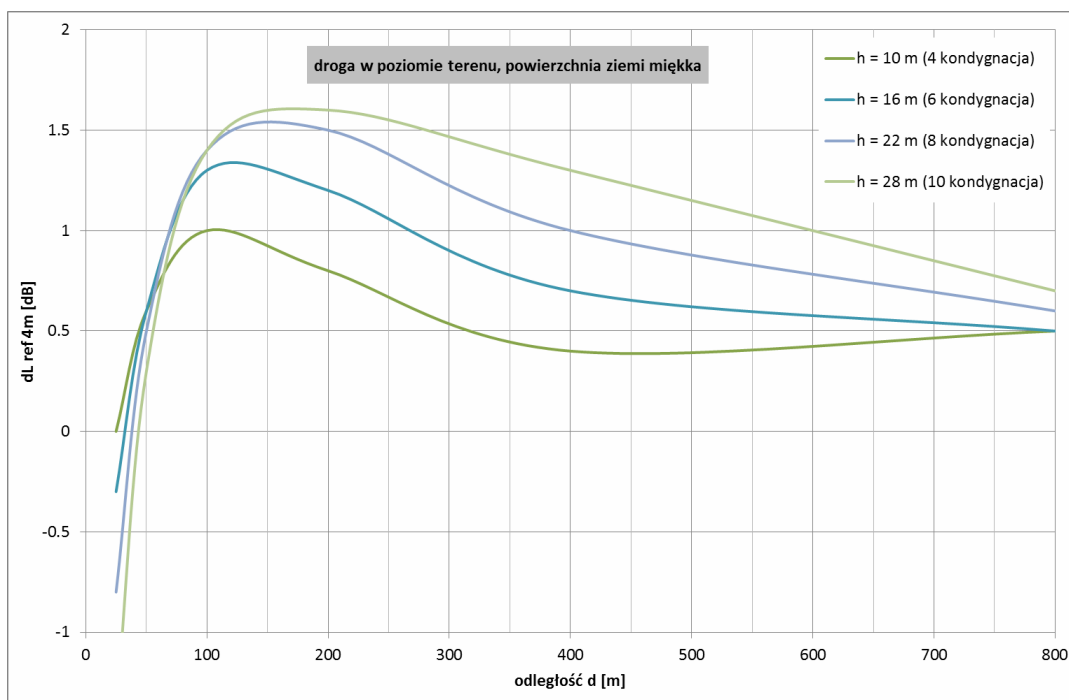
Rysunek 19: Różnice poziomu hałasu pomiędzy punktem na danej wysokości (poszczególne krzywe) a punktem na wysokości 4 metry – sytuacja dla drogi w poziomie terenu
