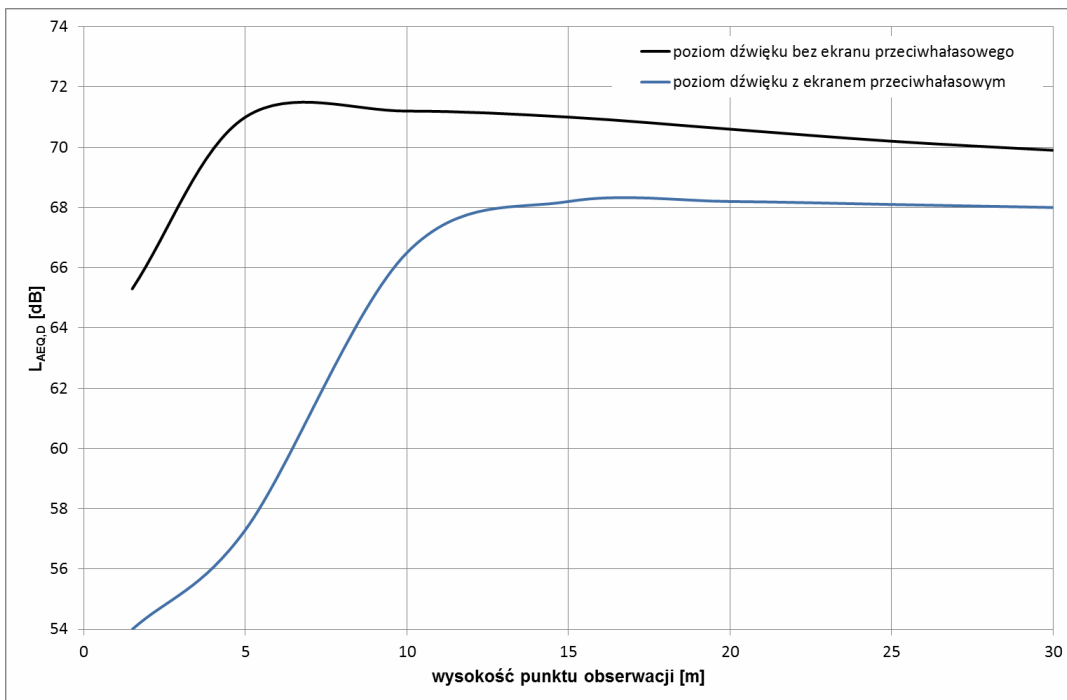
Rysunek 22: Zależność poziomu dźwięku od wysokości obserwatora dla drogi z ekranem przeciwhałasowym oraz bez ekranu przeciwhałasowego
