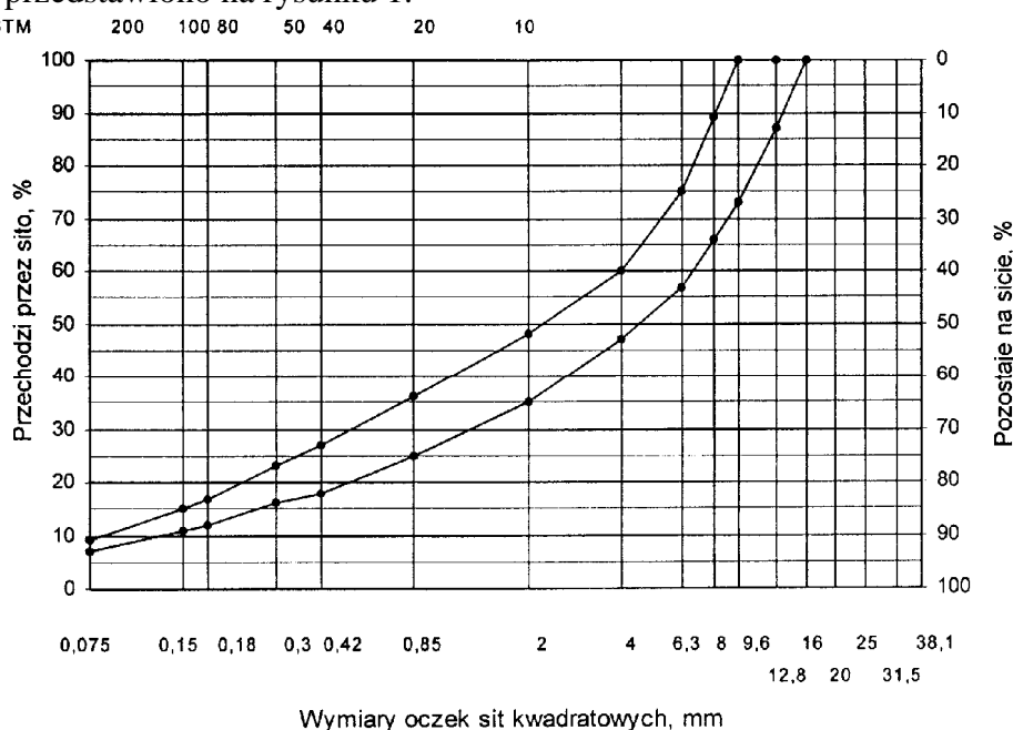
Rys. 1. Krzywa graniczna uziarnienia mieszanki mineralnej 0÷12,8 mm do warstwy ścieralnej z betonu asfaltowego dla KR 3
