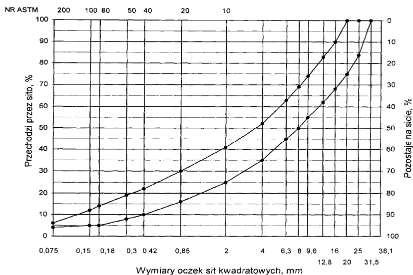
Rys. 2. Krzywe graniczne uziarnienia mieszanki mineralnej BA od 0 do 20 mm do warstwy wiążącej-wyrównawczej
