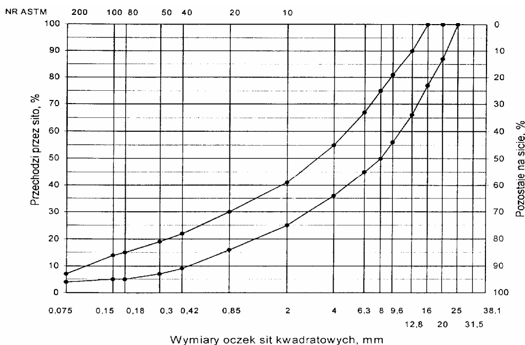
Rys. 2. Krzywe graniczne uziarnienia mieszanki mineralnej BA od 0 do 20 mm do warstwy wiążącej nawierzchni drogi o obciążeniu ruchem od KR3-4
