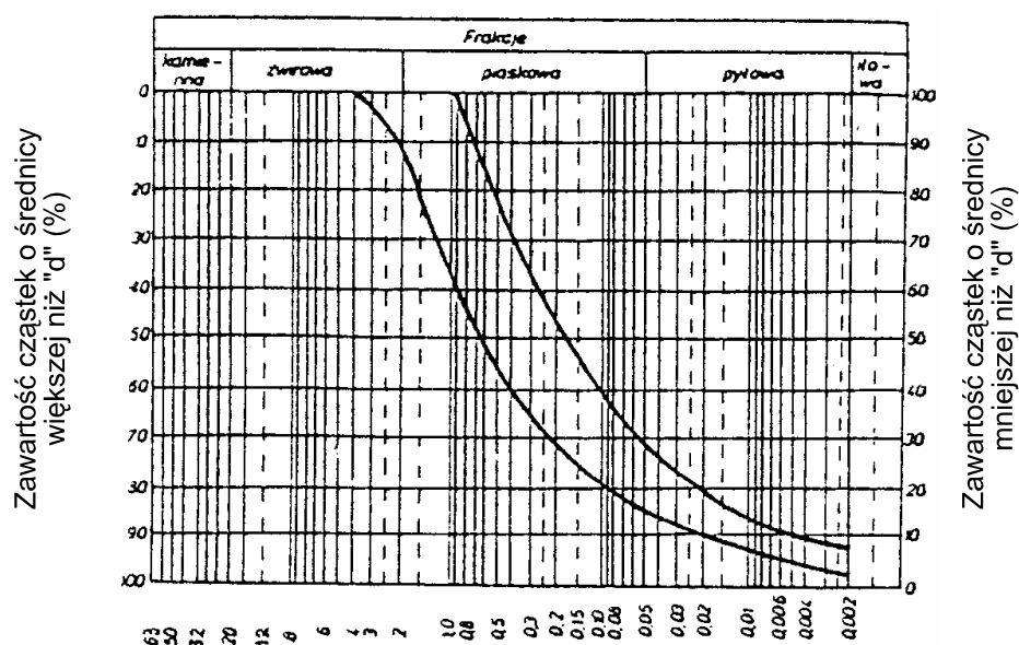
Rysunek 1. Obszar uziarnienia optymalnej mieszanki gliniasto-piaskowej
