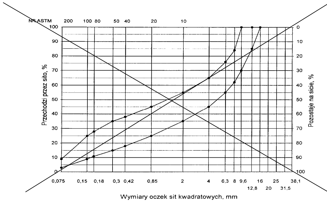
Rys. 1. Krzywe graniczne uziarnienia mieszanki mineralnej BA od 0 do 12,8 mm do warstwy wiążącej, wyrównawczej i wzmocniającej nawierzchni drogi o obciążeniu ruchem KR1 lub KR2
