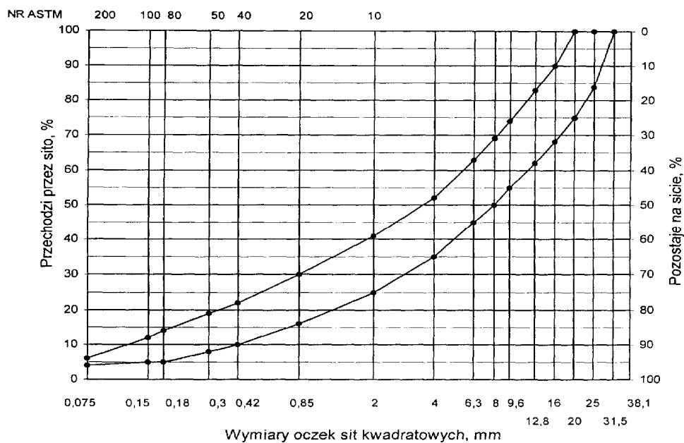
Rys. 2. Krzywe graniczne uziarnienia mieszanki mineralnej BA od 0 do 25 mm do warstwy wiążącej, wyrównawczej i wzmocniającej nawierzchni drogi o obciążeniu ruchem od KR3 do KR6
