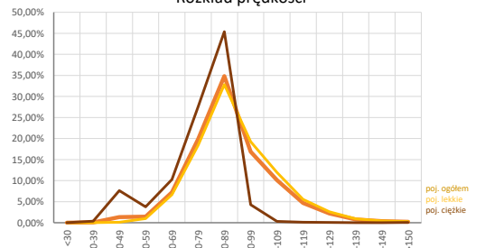
Rozkład prędkości
