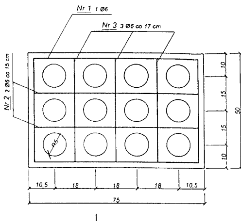
d) Płyta 0,75 × 0,50 × 0,10 m z otworami okrągłymi
