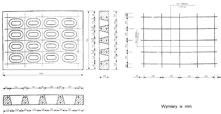
b) Płyta 1,0 × 0,75 × 0,125 m z otworami owalnymi
