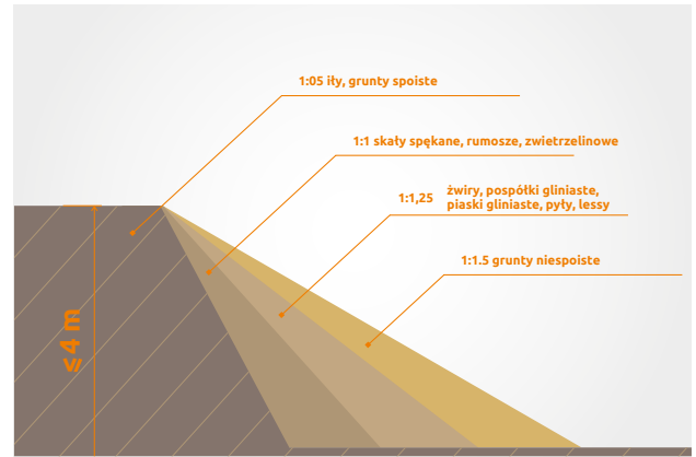
Rys. 6. Bezpieczne nachylenie skarp obudowami
