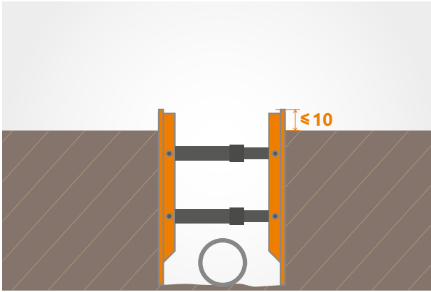
Rys. 1. Systemowa obudowa wykopu
