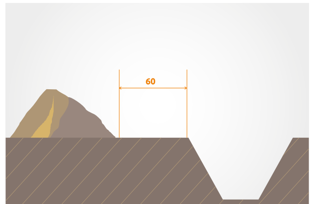
Rys. 2. Składowanie urobku
