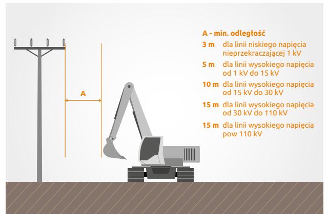
Rys. 6. Minimalna odległość prac od czynnej linii energetycznej w płaszczyźnie poziomej
