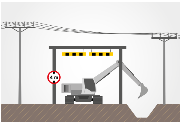
Rys. 5. Prace w bezpośrednim sąsiedztwie napowietrznych linii energetycznych
