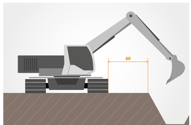
Rys. 4. Odległość koparki od wykopu
